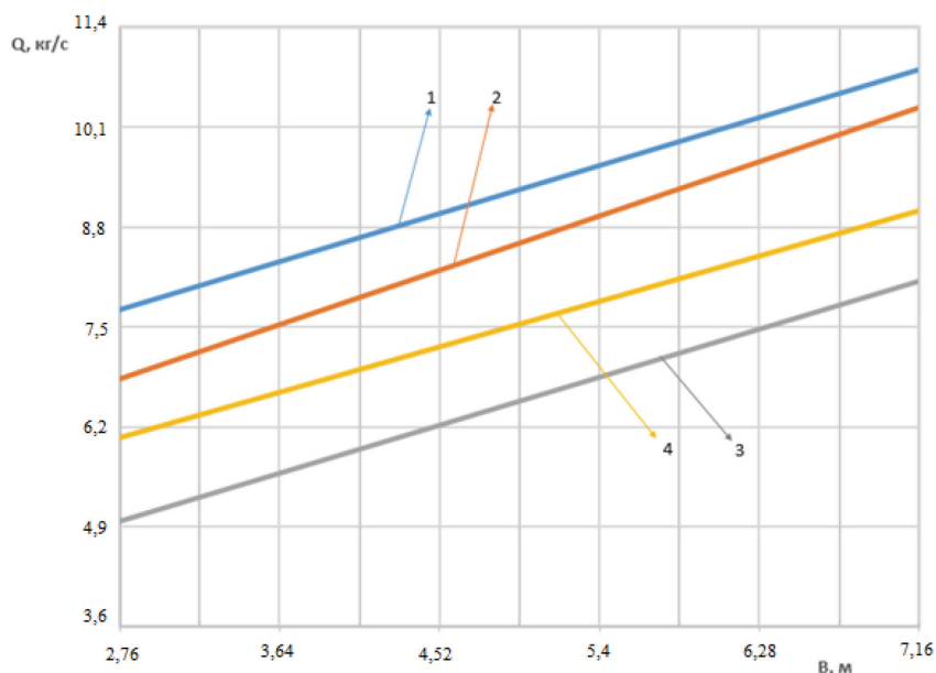
Рисунок 2 – Залежність подачі хлібної маси в молотарку від ширини захвату жнивarki та врожайності зерна Q = f(B; Y_z) :
