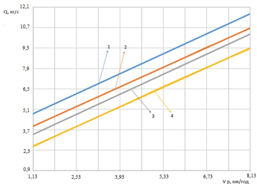
Рисунок 3 – Залежність подачі хлібної маси в молотарку від робочої швидкості комбайна та діаметра молотильного барабана Q = f(V_p; D_b) :
