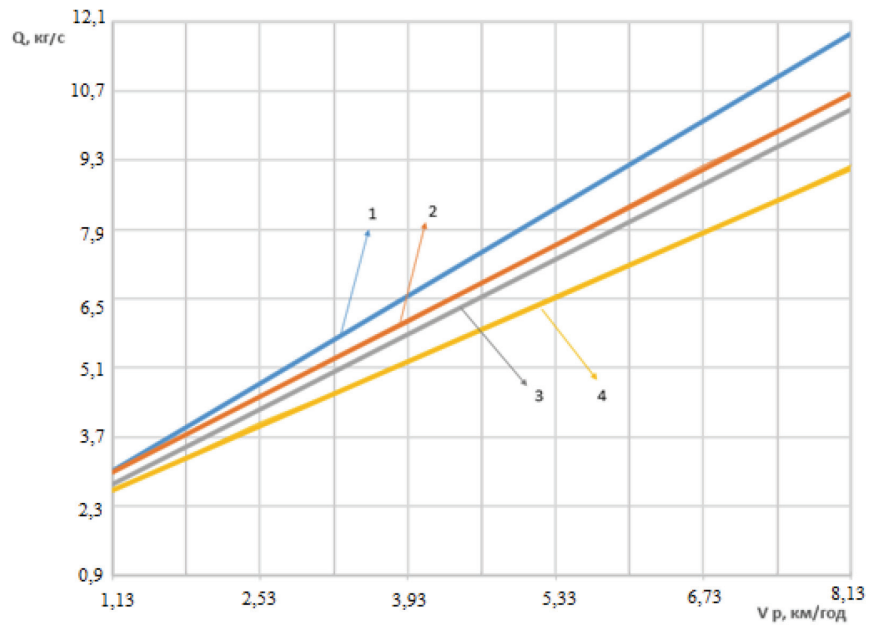
Рисунок 1 – Залежність подачі технологічної маси від робочої швидкості комбайна та ширини молотарки Q = f(V_p; B_m) : 1) B = 800 мм; 2) B = 1200 мм; 3) B = 1278 мм; 4) B = 1600 мм
