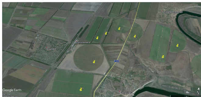
1 – дощувальні машини кругової дії; 2 - дощувальні машини кругової дії секторного поливу; 3 - дощувальні машини фронтальної дії; 4 - розподільчий канал Інгулецької зрошувальної системи Р-1
