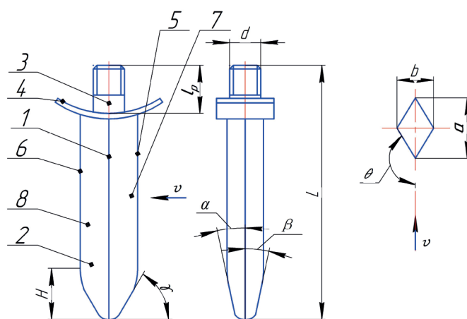
1 – основа; 2 – носок; 3 – хвостовик з різною; 4 – фіксатор; 5 – ребро робоче; 6 – ребро пасивне; 7 – грань робоча; 8 – грань пасивна; \alpha , \beta – кути загострення (конфігурації) носка; \gamma – кут входження носка; \theta – кут розкриття борозни; a – довжина перерізу профіля основи; b – ширина перерізу профіля основи; H – висота носка
