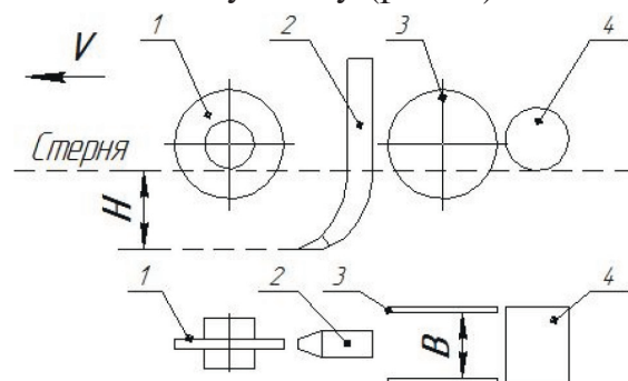
1 – передній диск; 2 – долото; 3 – відрізнні бокові диски; 4 – прикочувальний коток. B – відстань між відрізнними боковими дисками; H – глибина обробітку долотом; V – швидкість руху МТА
