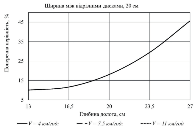
Рисунок 7 – Залежність поперечної нерівності від глибини обробки долотом H за відстані між боковими відрізними дисками B = 20 см
