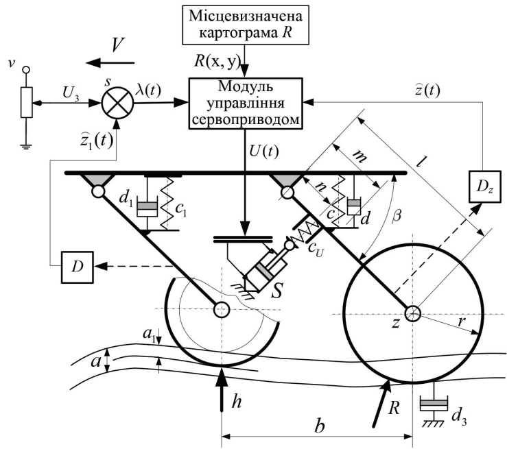
Рисунок 2 – Сошниковая система з автоматизованою системою корекції положення вдавлювального диска
