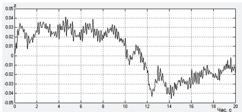
Рисунок 4 – Графік реалізації глибини ходу вдавлювального диска
